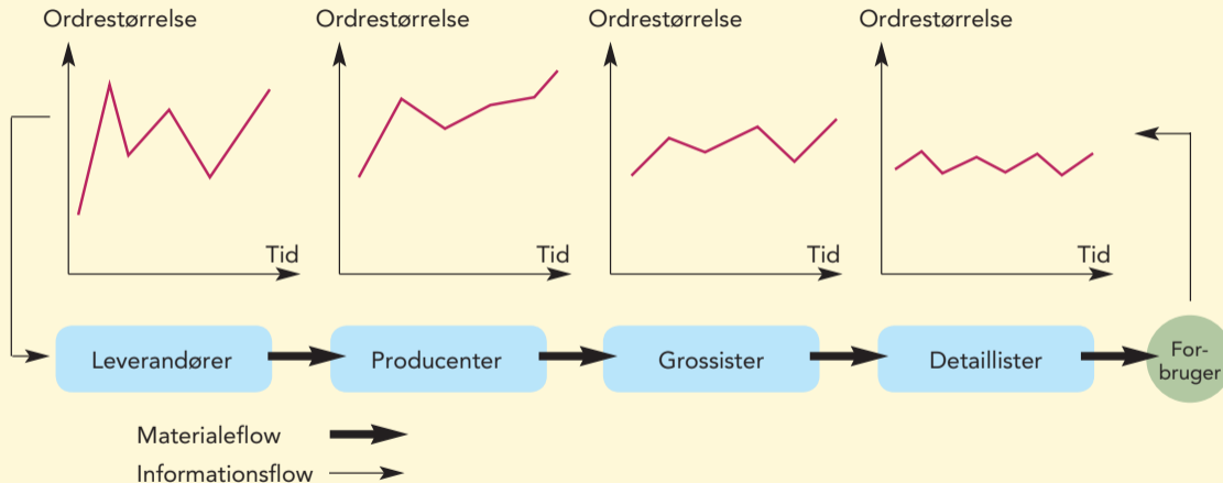
Fig. 1.4 Princippet i Forrestereffekten.
