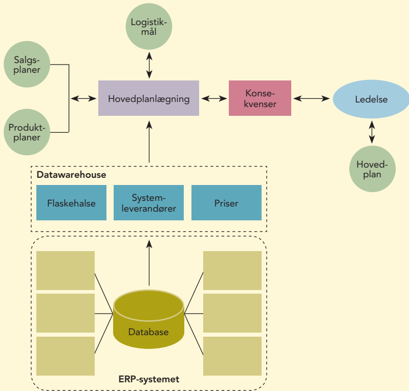
Fig. 8.6 Princippet i et DSS-system til hovedplanlægning.
