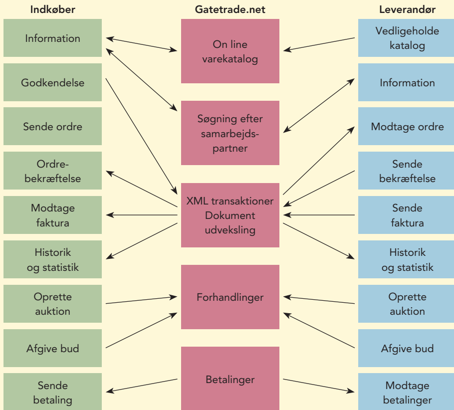
Fig. 8.12 Eksempel på e-procurement hos Gatetrade.
