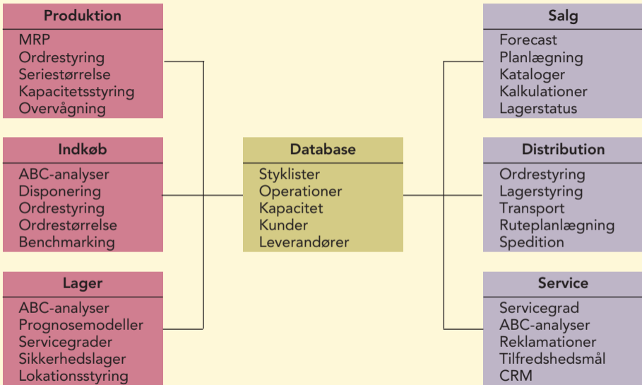
Fig. 8.4 Eksempler på funktioner i forskellige moduler i ERP-systemer.
