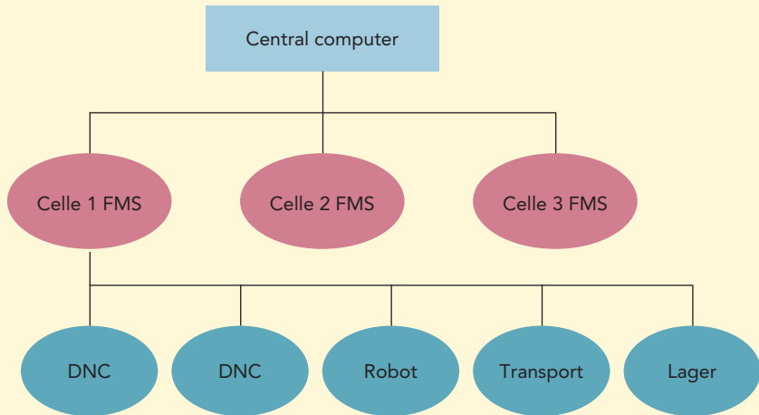
Fig. 8.13 Princippet i FMS systemer.
