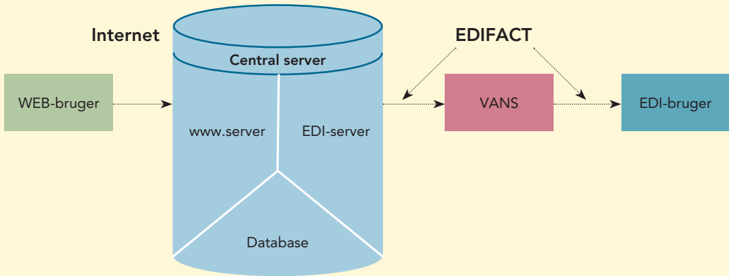
Fig. 8.18 Eksempel på anvendelse af Web-EDI.
